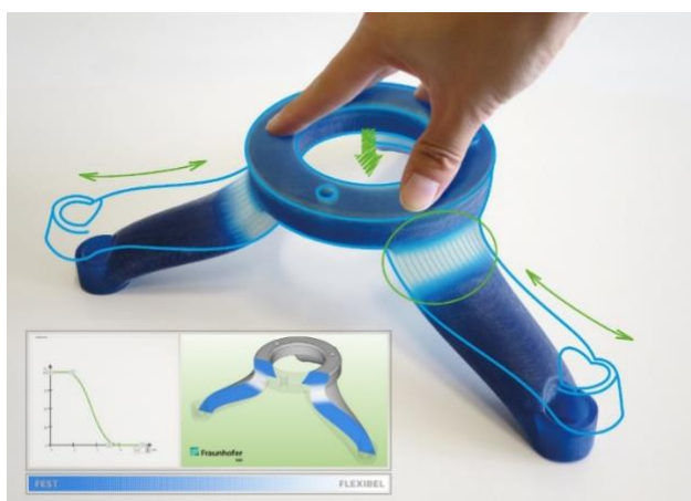
Abb. 3: FGM-Bauteil „Kamerastativelement“ mit Kombination aus hartem (blau) und elastischen Material (weiß) und gradierten Übergängen dazwischen.
